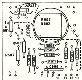
POTENTIOMETER PLAAT PLAQUE DE POTENTIOMÈTRE KY 595
